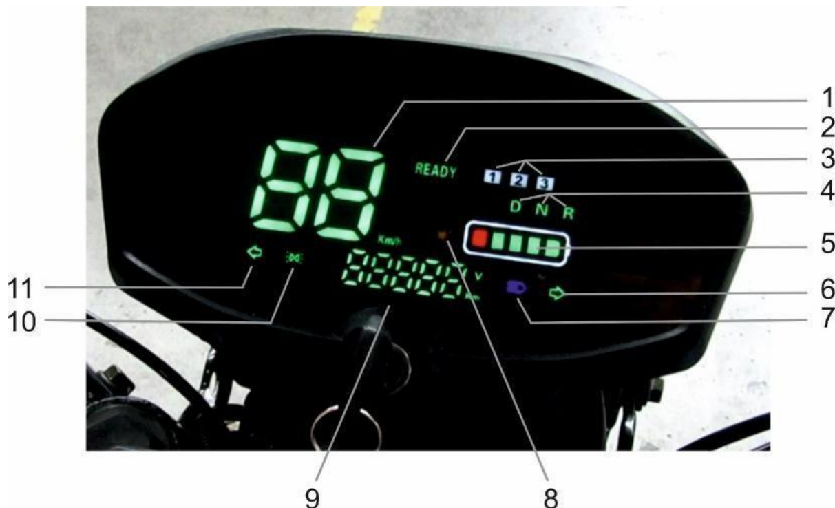
Figura 1-1 Afișaj bord
