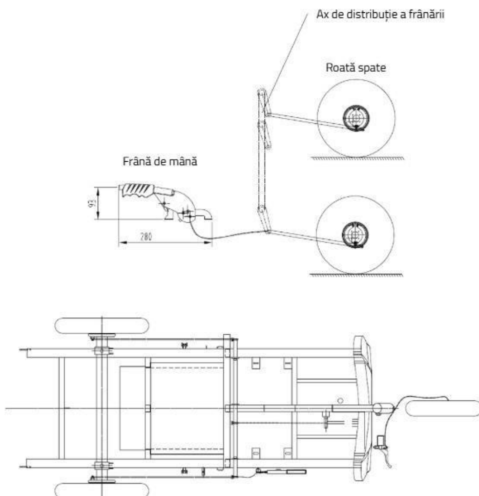
Figura 1-6 Frâna de parcare
