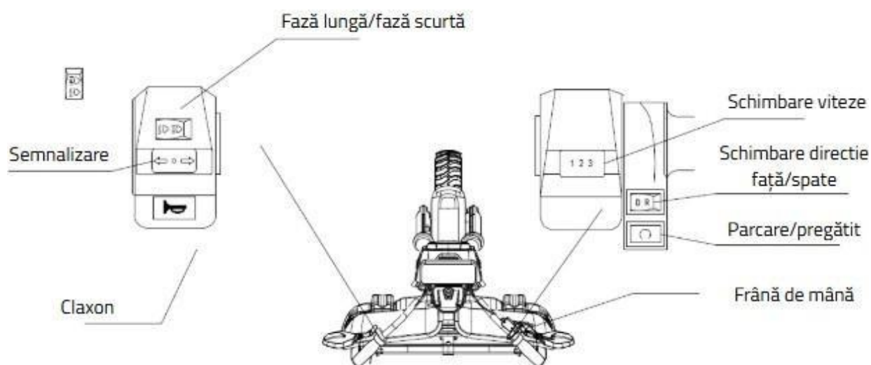
Mâner stânga
