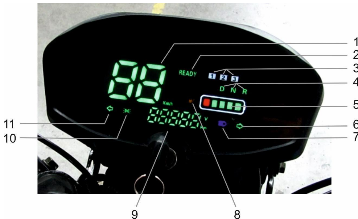
Figura 1-1 Afișaj bord
